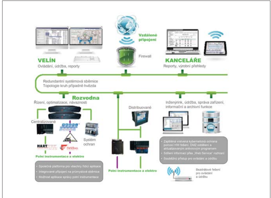
Schéma Valmet DNA
