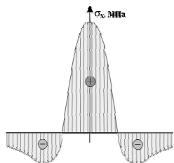
Kontrola svarů – typické rozložení zbytkových napětí
